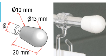
Tappo antinfortunio in gomma bianca. Safety end cap in white rubber.
