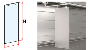
Busta trasparente antiriflesso (spessore 0,4 + 0,4 mm). Transparent antiglare pocket (0,4 + 0,4 mm thickness).
